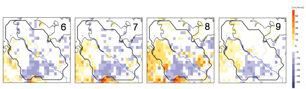
Abbildung 44 Differenz der Evapotranspiration [mm/Monat] (LUCbewmax-REFbewmax) in der MRH für die Monate Juni-September im Jahr 2003
