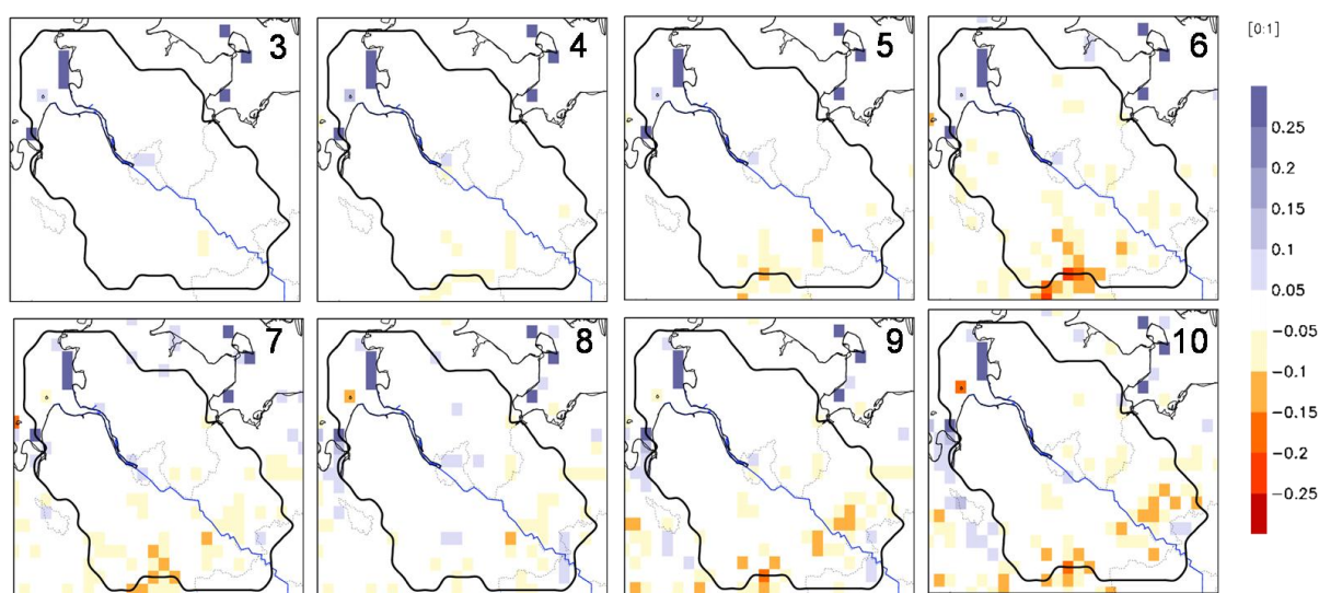
Abbildung 39 Differenz der 2 m-Temperatur (LUC-REF) in der MRH für die Monate März-Oktober im Jahr 2002
